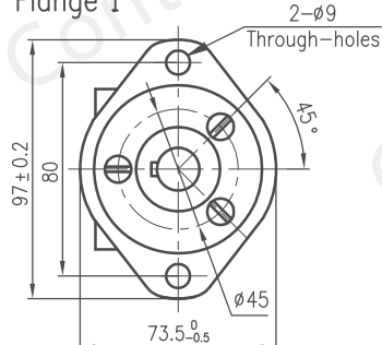
Flange I
